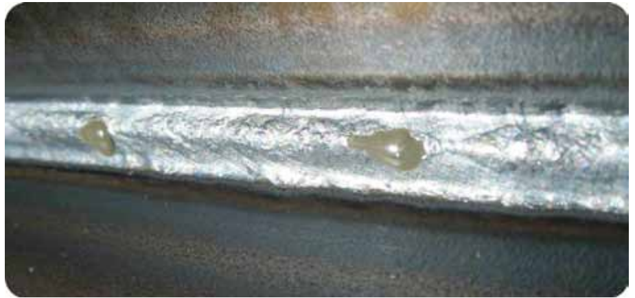
Kuva 3. CMT, materiaali 3 mm S355J2H, lisäaine 1,0 mm G3Si1, suojakaasu 100 % CO 2 , hitsausnopeus 100 cm/min.
